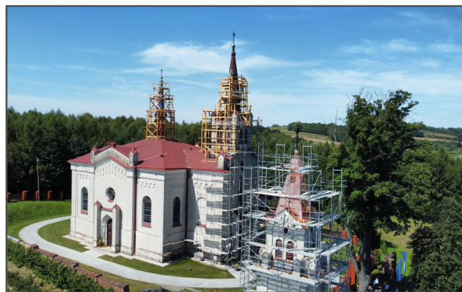
Wymiana pokrycia dachowego na budynku zabytkowego Kościoła w Batorzu Pierwszym
