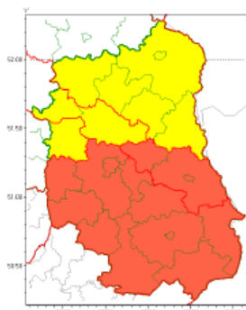
Intensywne opady śniegu 2021-02-07 06:59
